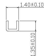
SEC:D-D
